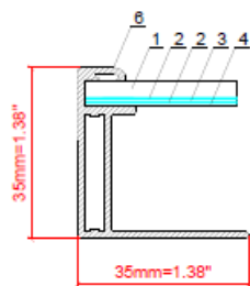
Section A-A 8:1
