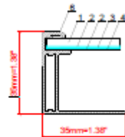
Section A-A 8:1
